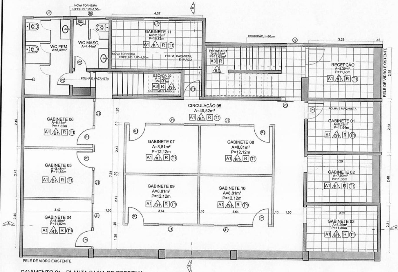
PAVIMENTO 01 - PLANTA BAIXA DE REFORMA esc 1:75
